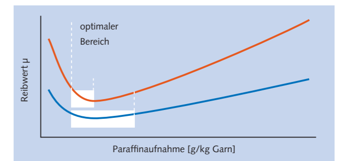
Die Paraffinierungskurve zeigt das Verhältnis zwischen Reibwert und Aufnahme bei verschiedenen Materialien wie Chemiefaser oder Baumwollgarne. Der weiße Bereich zeigt das optimale Verhältnis.
