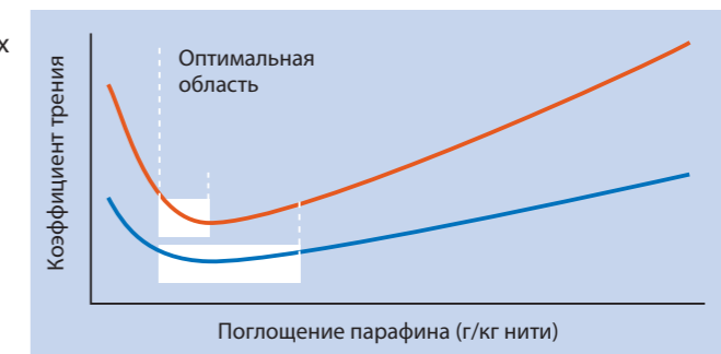
Кривая парафинизации показывает соотношение между коэффициентом трения и поглощением парафина разными материалами, такими как ■ синтетические волокна или ■ хлопковая пряжа. Белая область указывает на оптимальные соотношения.
